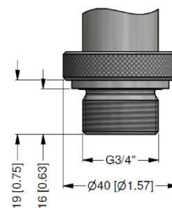
G3/4" semi-flush DIN 3852 (0.6 bar ≤ p N ≤ 60 bar gauge)
