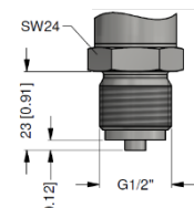
G1/2" EN 837
