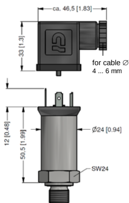
ISO 4400 (IP 65)
