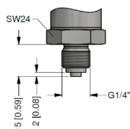
G1/4" EN 837
